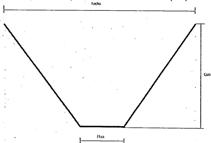
Figura 4: geometría y dimensiones de canales (Trapezoidal).
